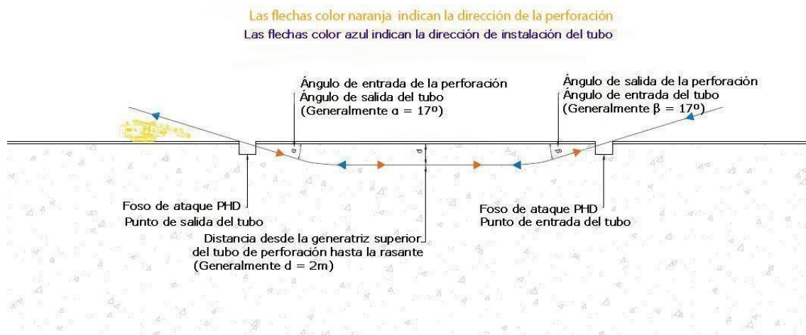
Figura 6. Esquema de perforación e instalación del tubo cruzamiento en la carretera.
